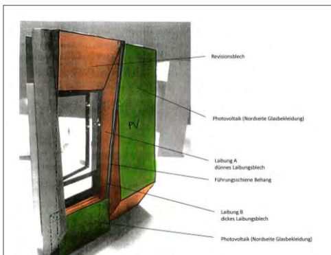
Entwurf, Übersicht
